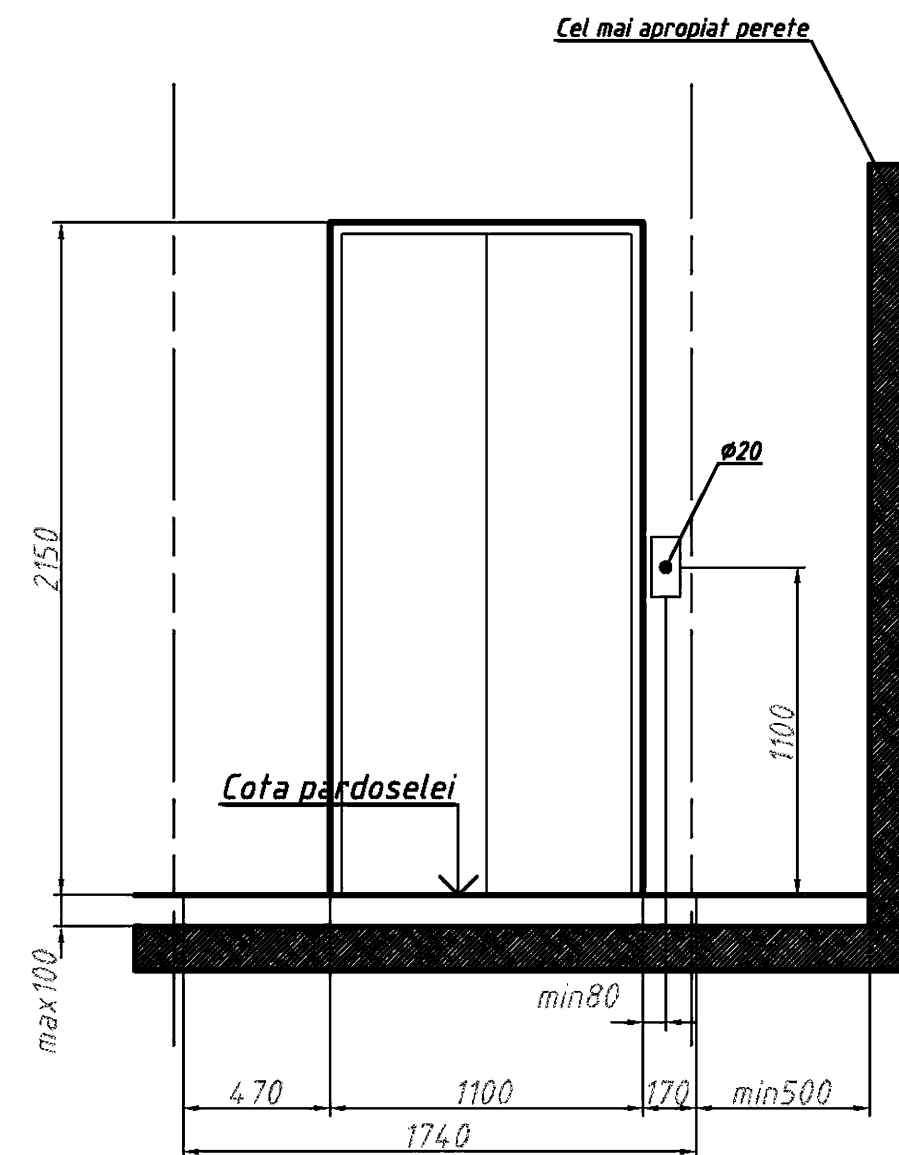
Etajele intermediare
